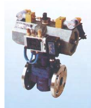
X643W-10P 气动二通旋塞阀
